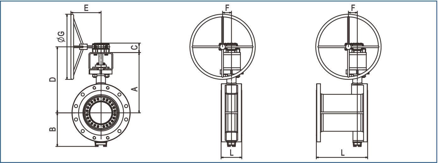
法兰端
