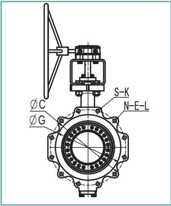
凸耳式
