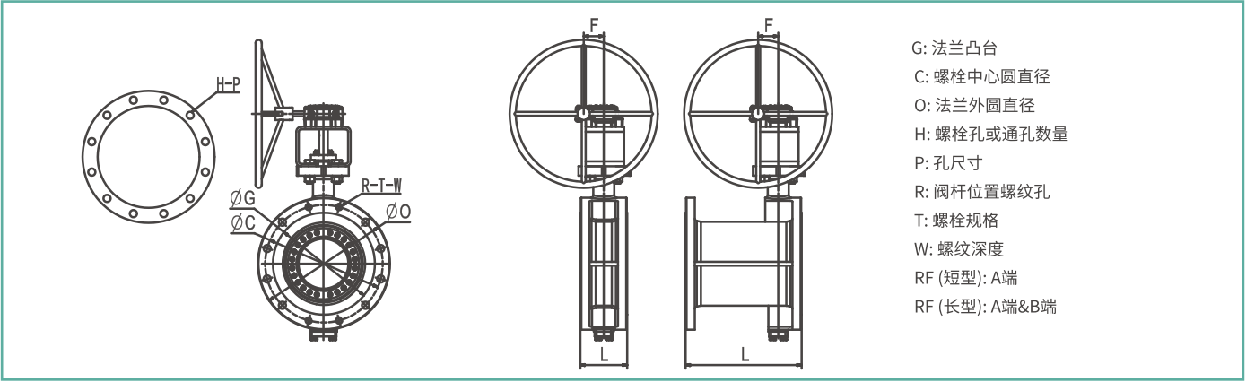
Class 150 (双法兰) 双法兰
