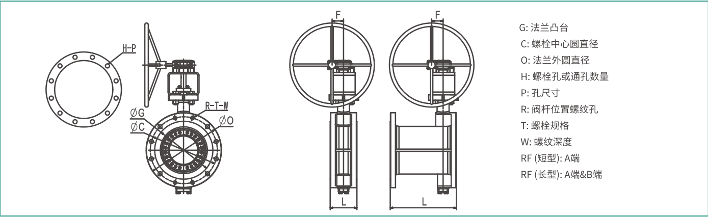
Class 900 (双法兰) 双法兰
