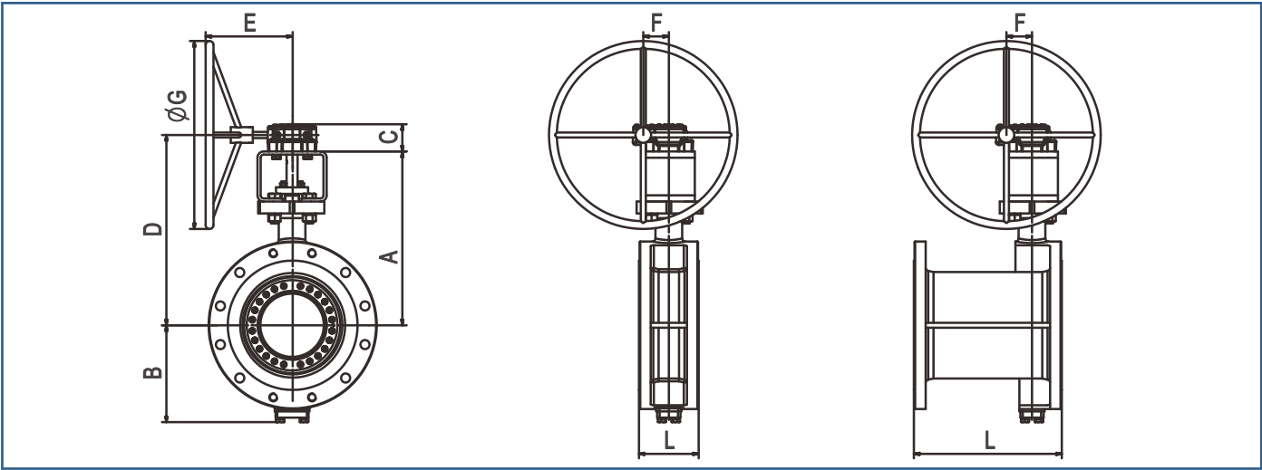
法兰端
