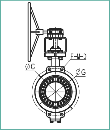
对夹式
